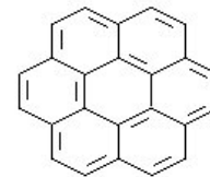
Coronene
